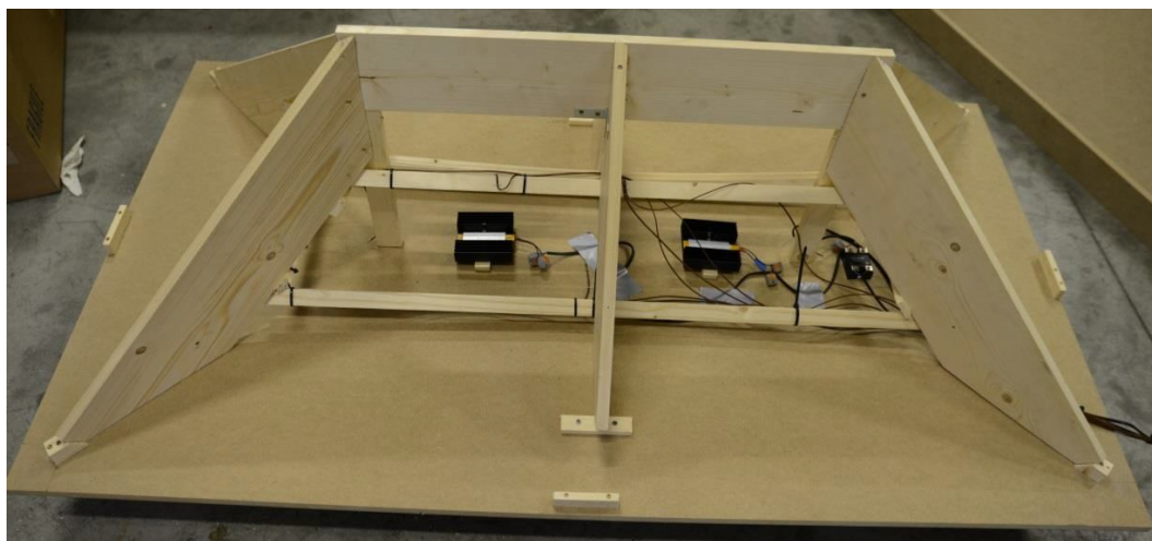
Rysunek 2 - Podstawowa konstrukcja drewniana i system ogrzewania
